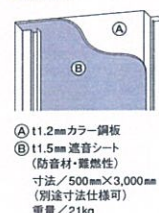
A) 11.2mm カラー鋼板 B) 11.5mm 遮音シート (防音材・難燃性) 寸法/500mm×3,000mm (別途寸法仕様可) 重量/21kg
