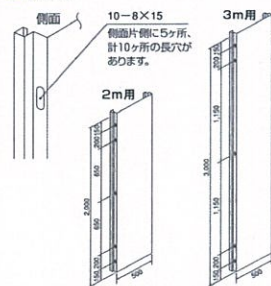
寸法/500mm×2,000mm 2型 14kg (防音材あり) 寸法/500mm×3,000mm 2型 21kg (防音材あり)
