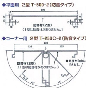
A) 11.2mm カラー鋼板 B) 11.5mm 遮音シート (防音材・難燃性) 寸法/500mm×3,000mm (別途寸法仕様可) 重量/21kg
